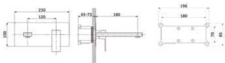
Ref. 3028 Grifo empotrable de lavabo ORION CROMO Puntos 139
